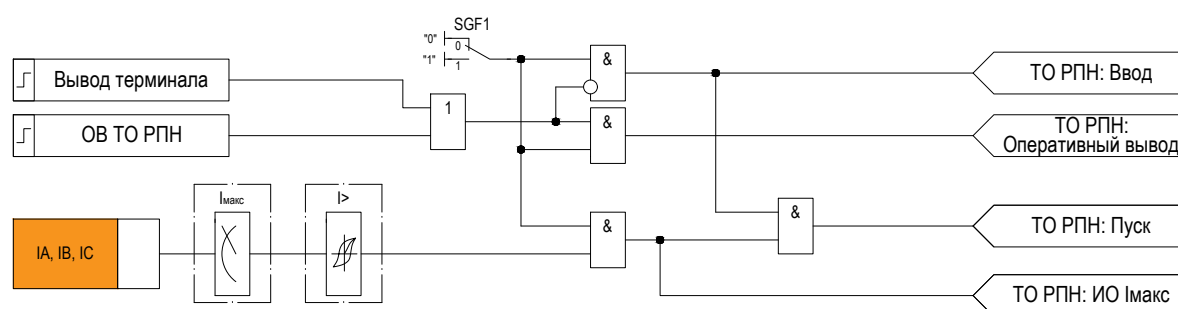
Рисунок 2.10 – Функциональная схема логики ТО РПН
